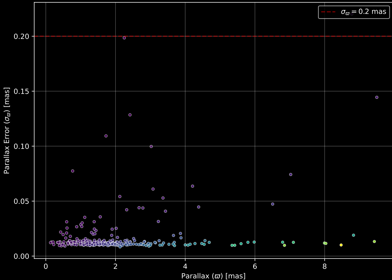
GALAH DR4 Field: [6918] Parallax Quality (n= 294)
