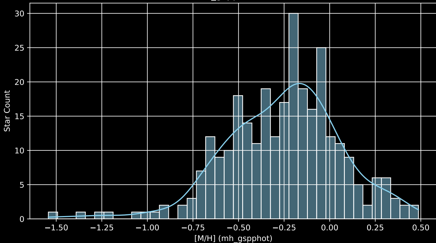
GALAH DR4 Field: [6918] [M/H] (mh_gspphot) (n= 291)
