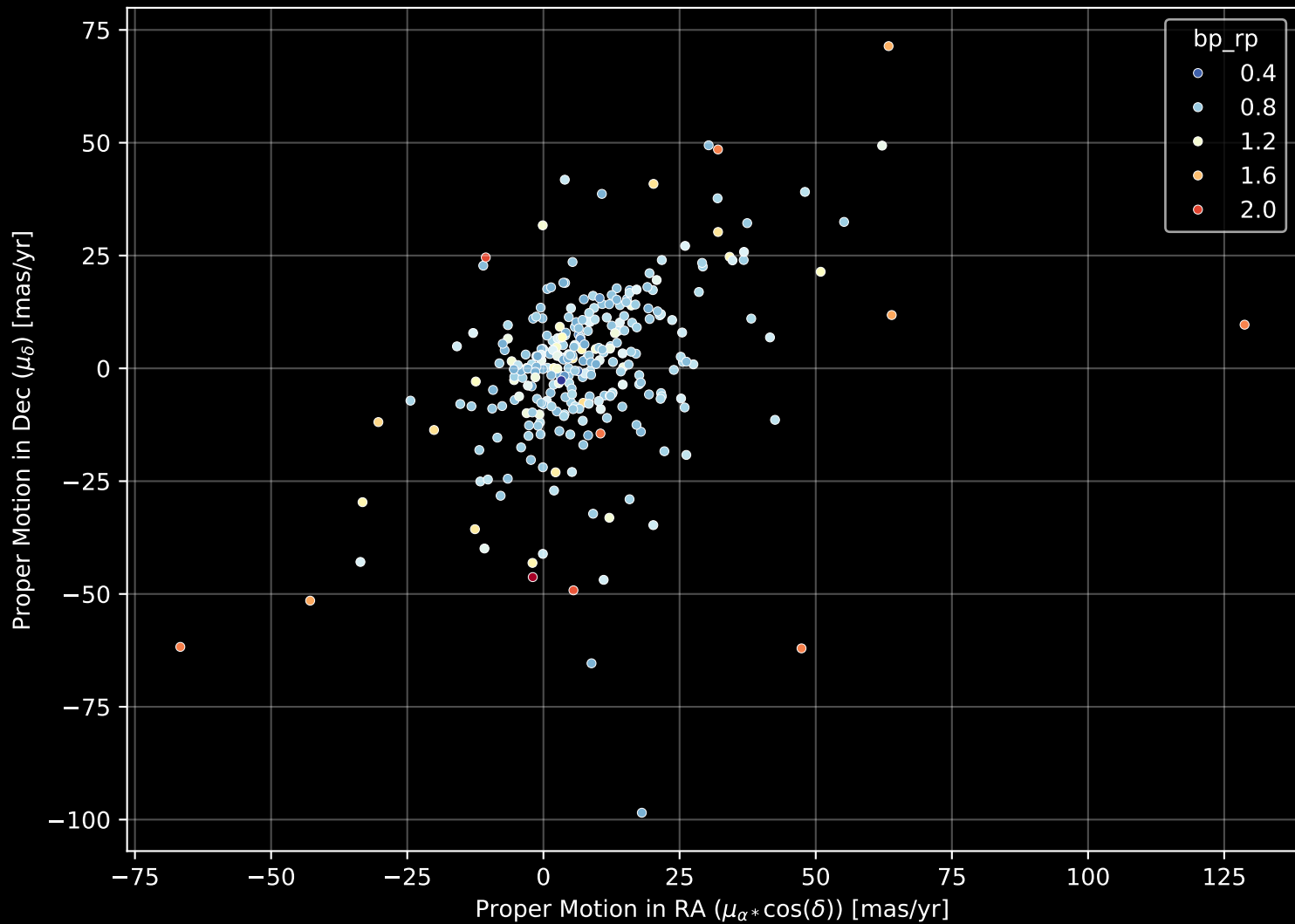
GALAH DR4 Field: [6918] Proper Motion Diagram (n= 294)
