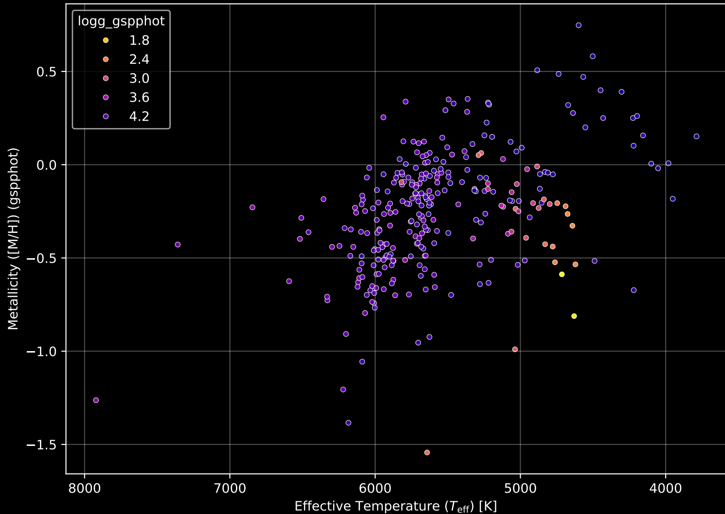
GALAH DR4 Field: [6918] Stellar Population Parameters (n= 294)
